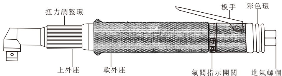
規格一覽表(弯头)
